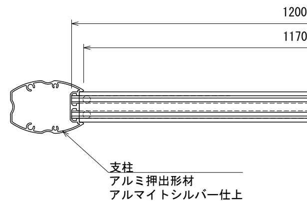
【平面図 S=1:5】
