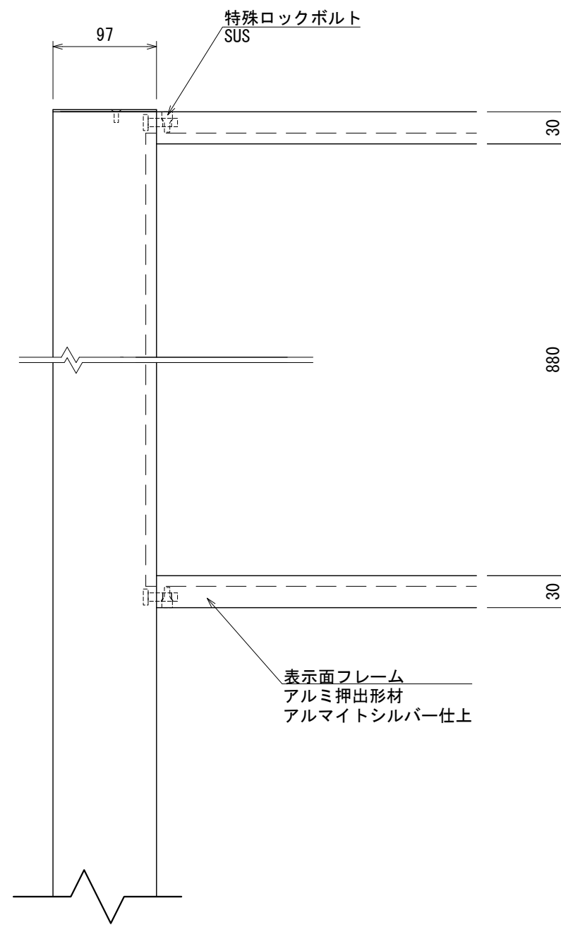
【正面図 S=1:5】
