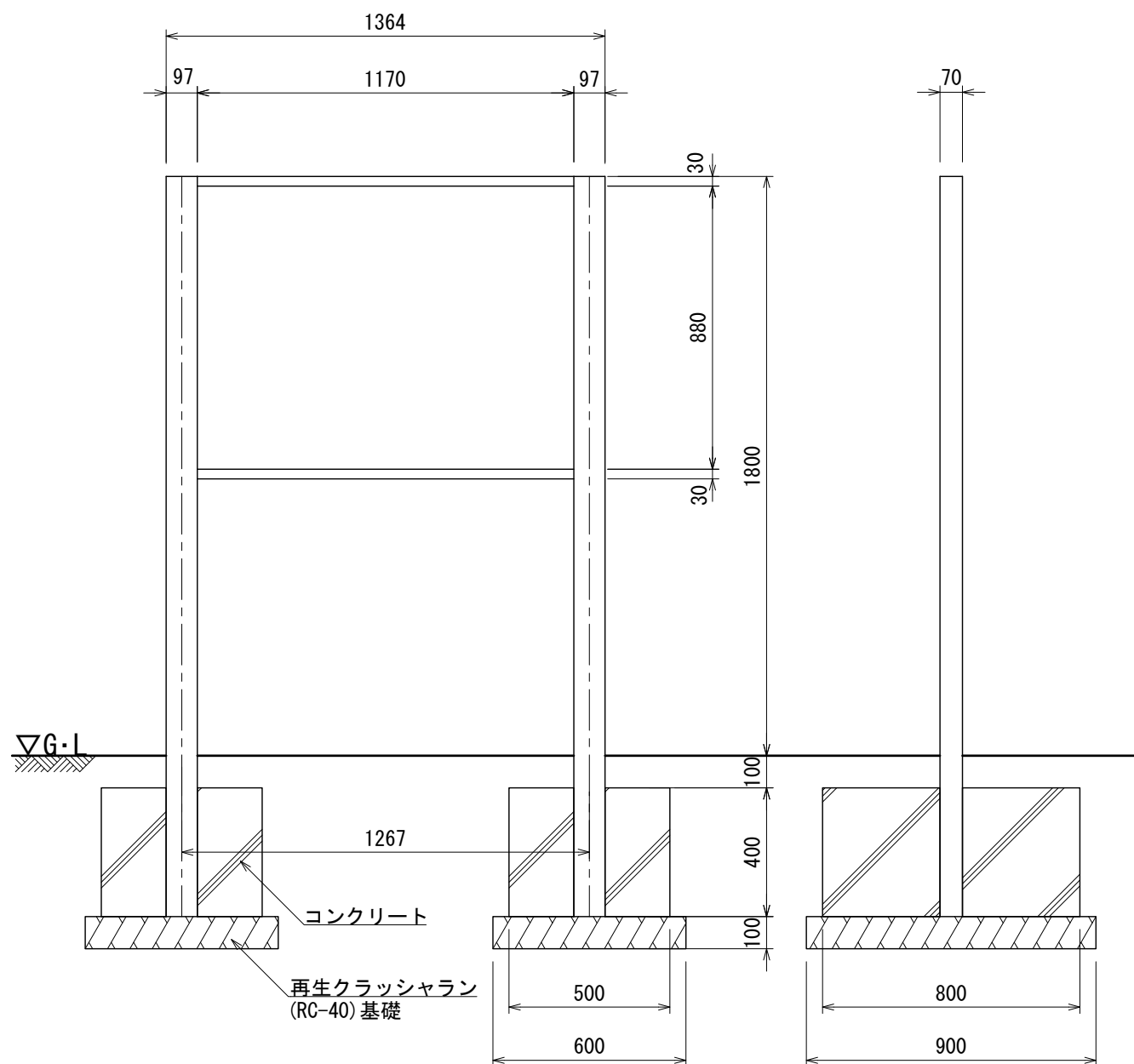
【正面図】
