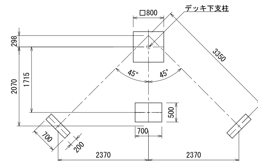
基礎伏図
