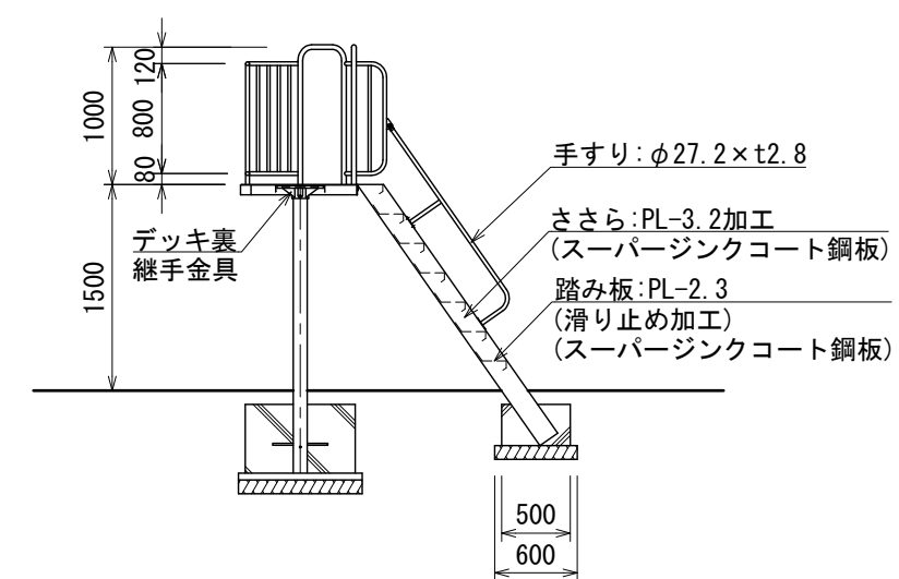
A-A断面図
