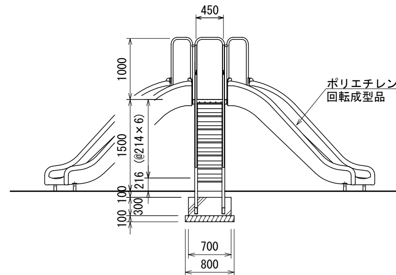
正面图
