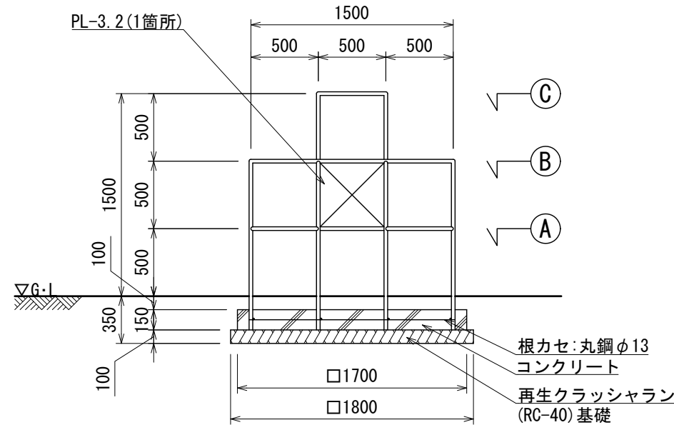
立面図
