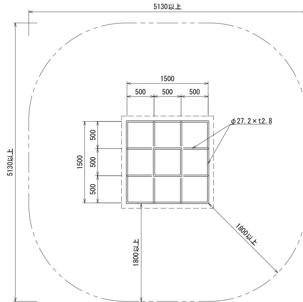
平面図
