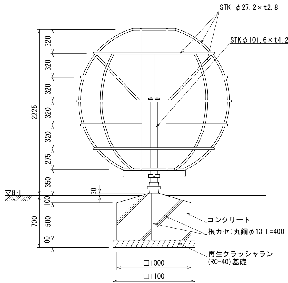
立面図
