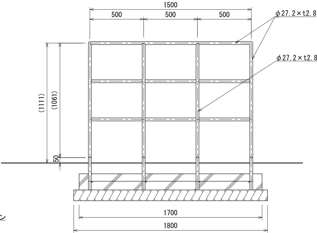
安全領域図 S=1:100
