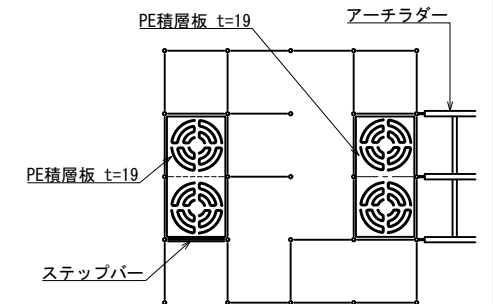
B断面図
