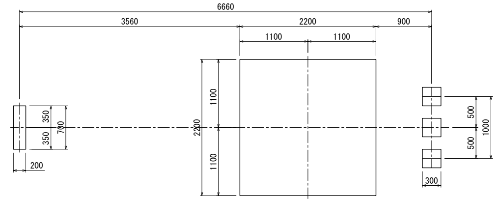
基礎伏図
