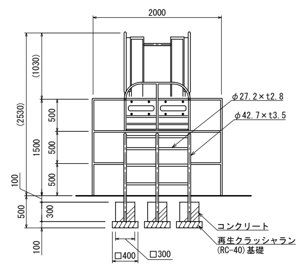
背面図
