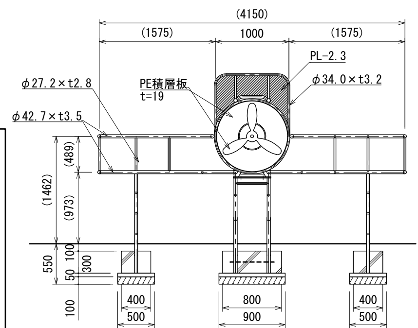
A矢視図
