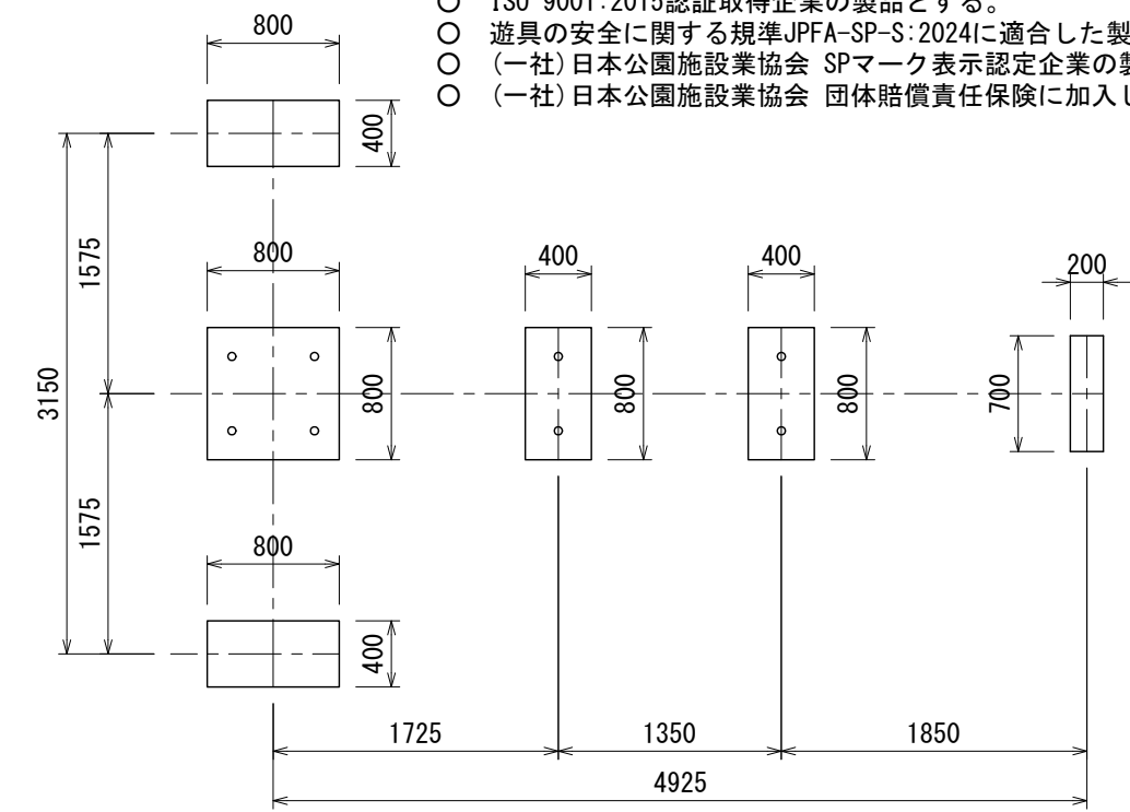
基礎伏図
