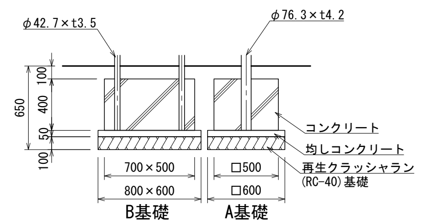
基礎詳細図
