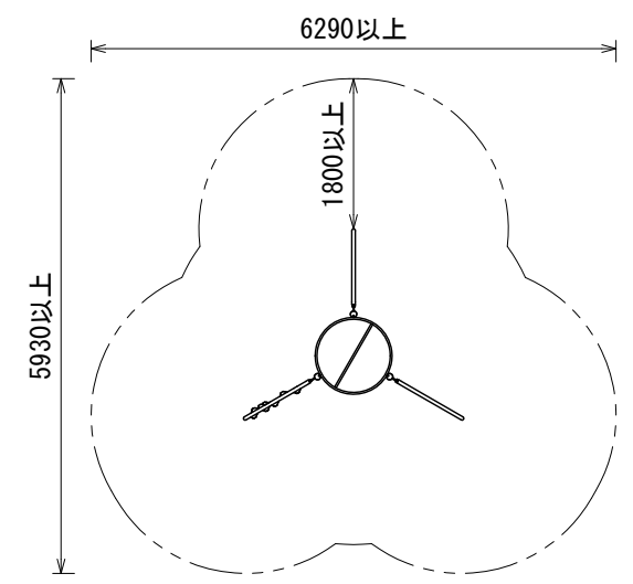
安全領域図 S=1:100
