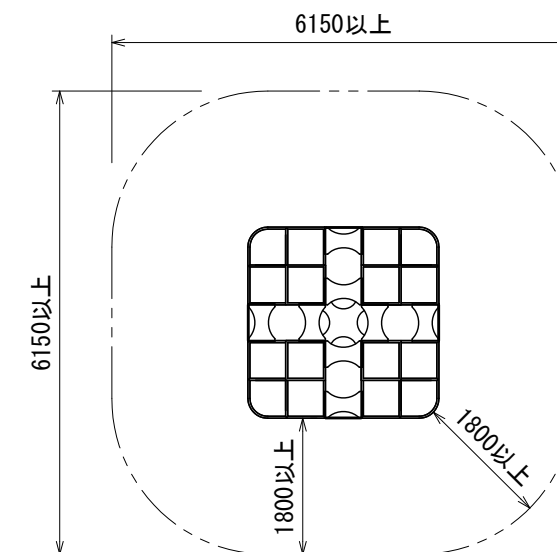
安全領域図 S=1:100
