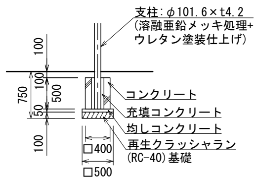
踊り場支柱部基礎図
