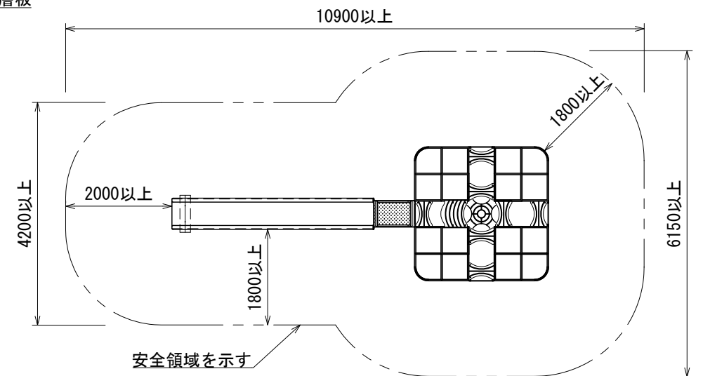
安全領域図 S=1:100
