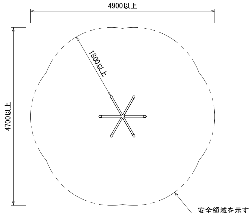
安全領域図 S=1:60
