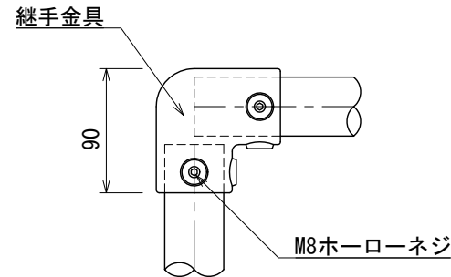
継手金具部詳細 S=1:5
