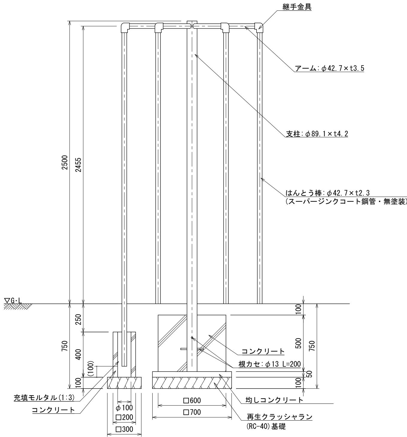
立面図
