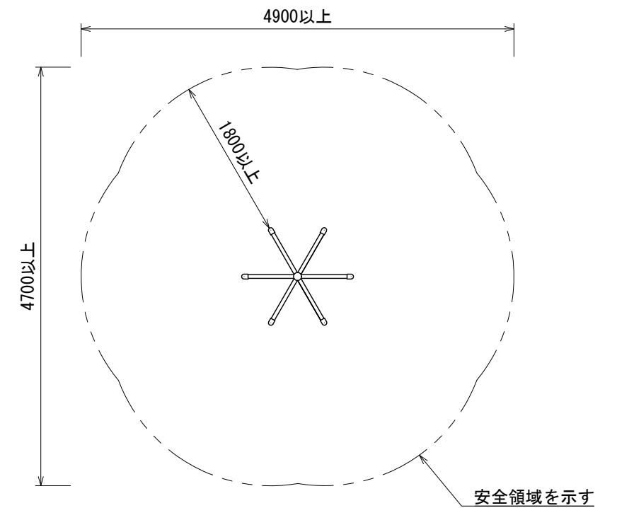
安全領域図 S=1:60
