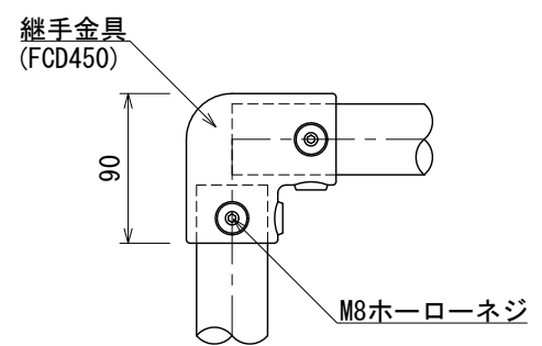
継手金具詳細 S=1:5
