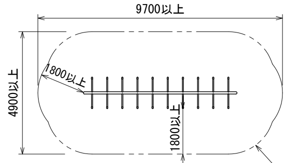
安全領域図 S=1:150
