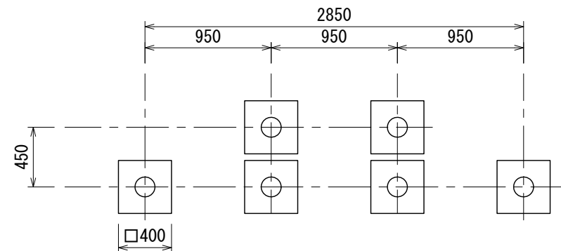
基礎伏図
