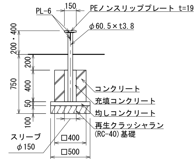
基礎詳細図 S=1:30
