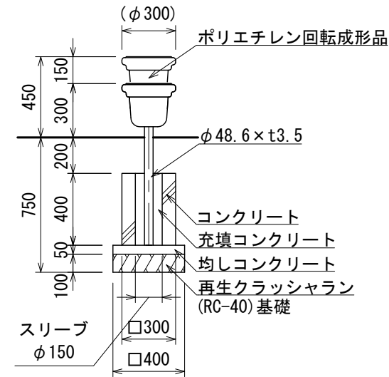
B'1基礎詳細図
