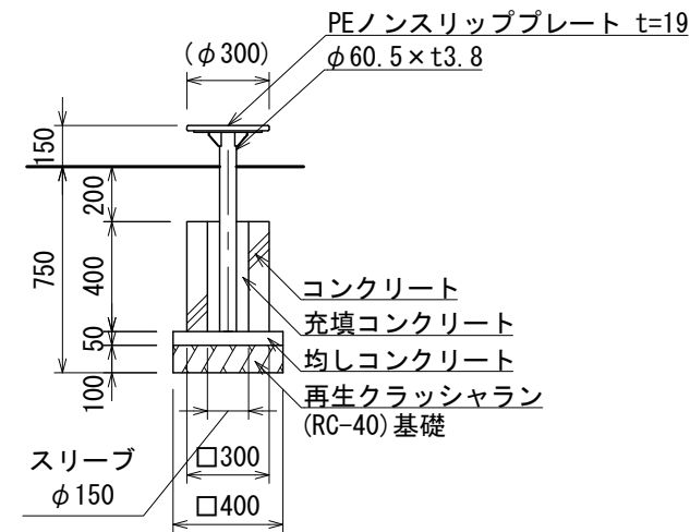
B'2基礎詳細図
