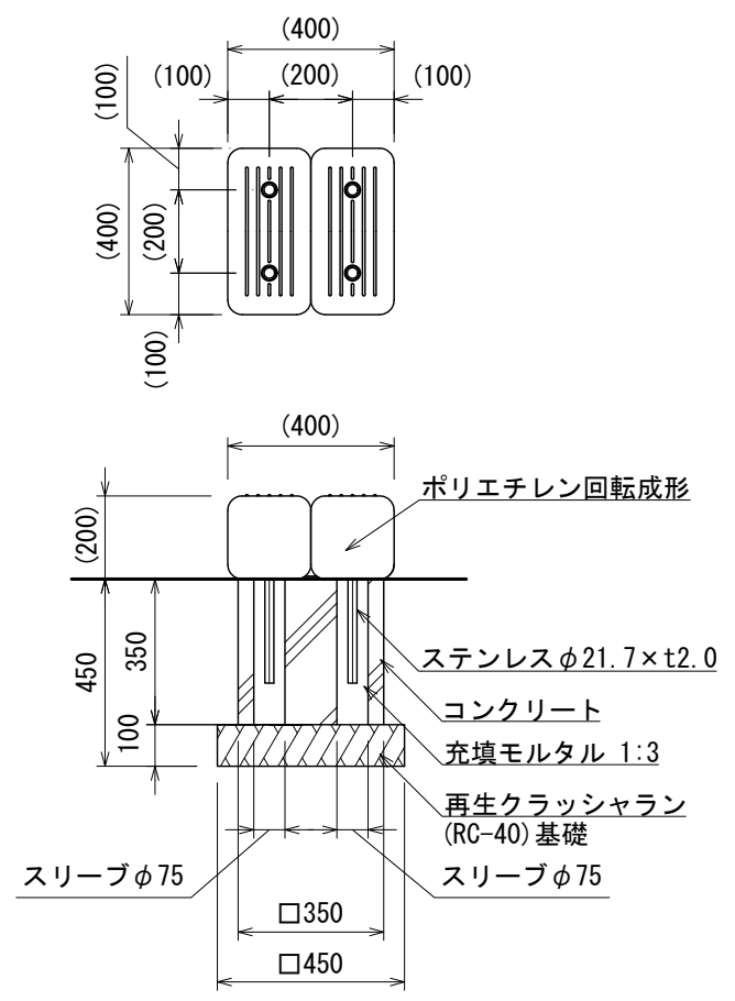
詳細図 S=1:20 H200 (2列)
