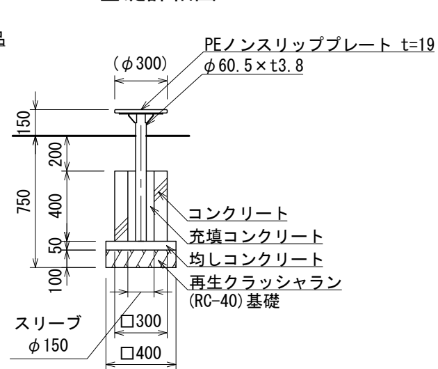
B' 2基礎詳細図
