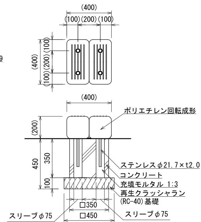
C' 基礎詳細図
