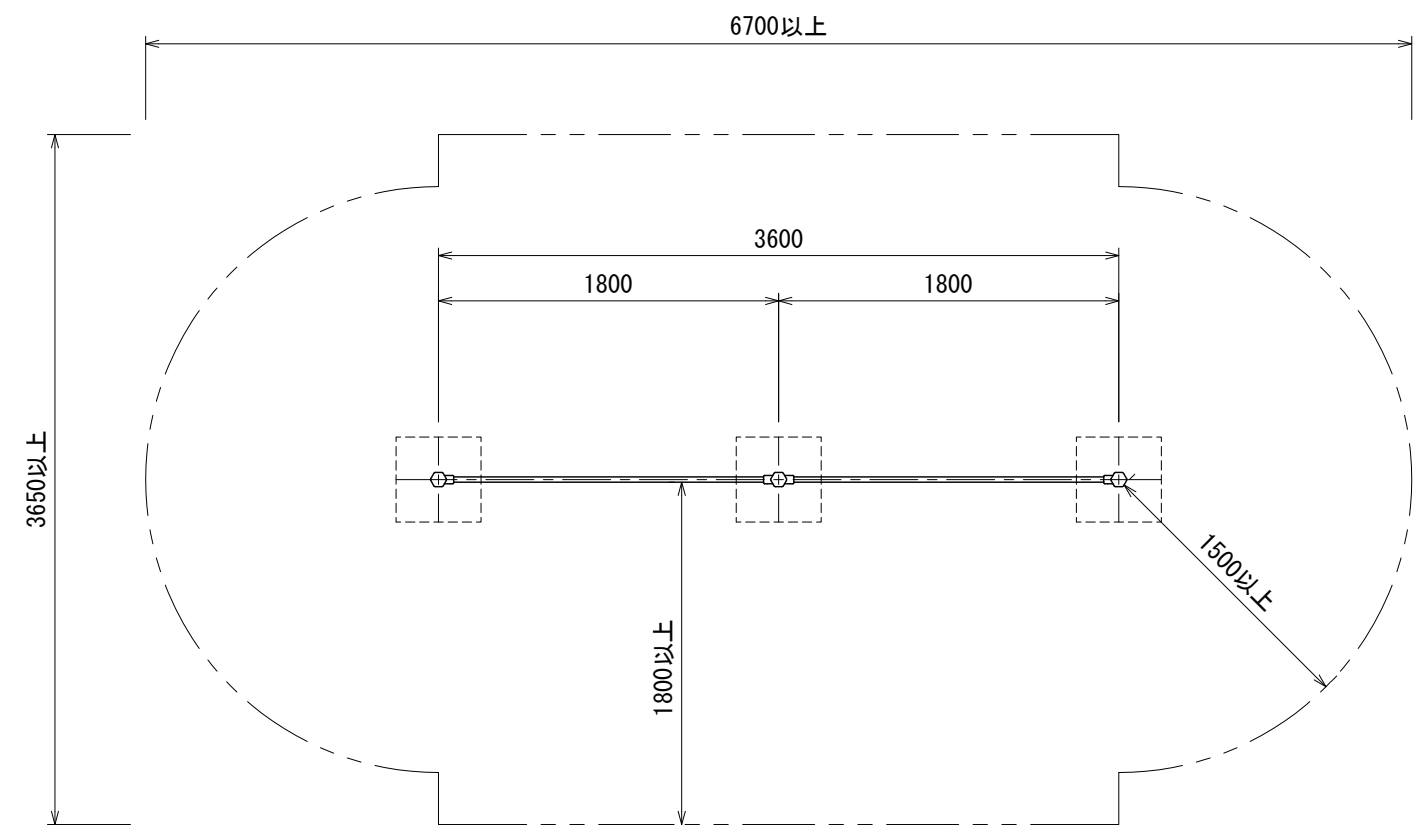
平面図
