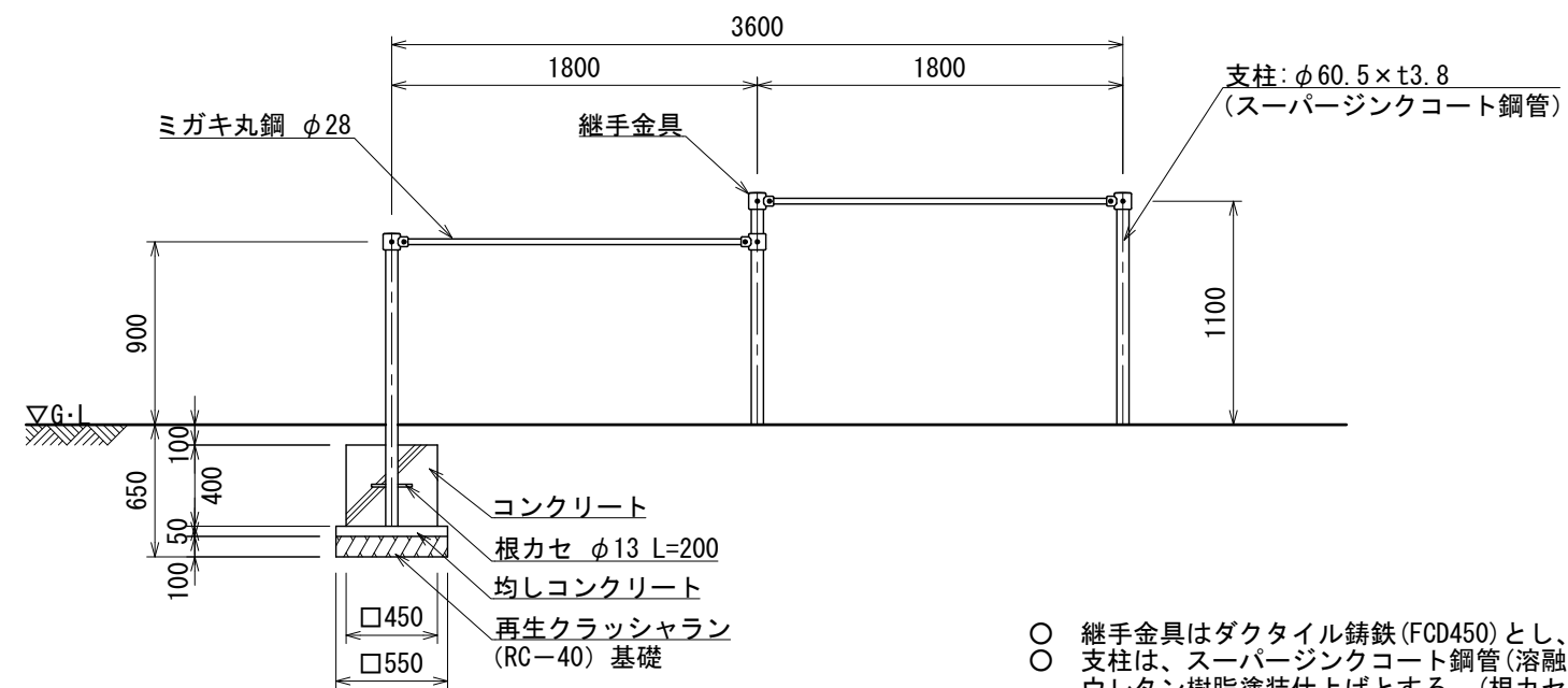
立面図
