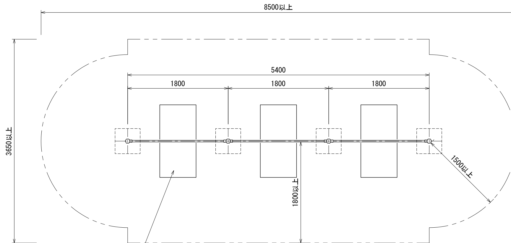
平面図
