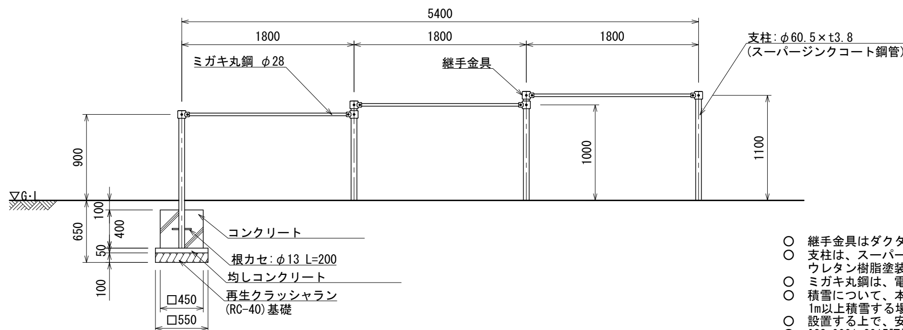
立面図
