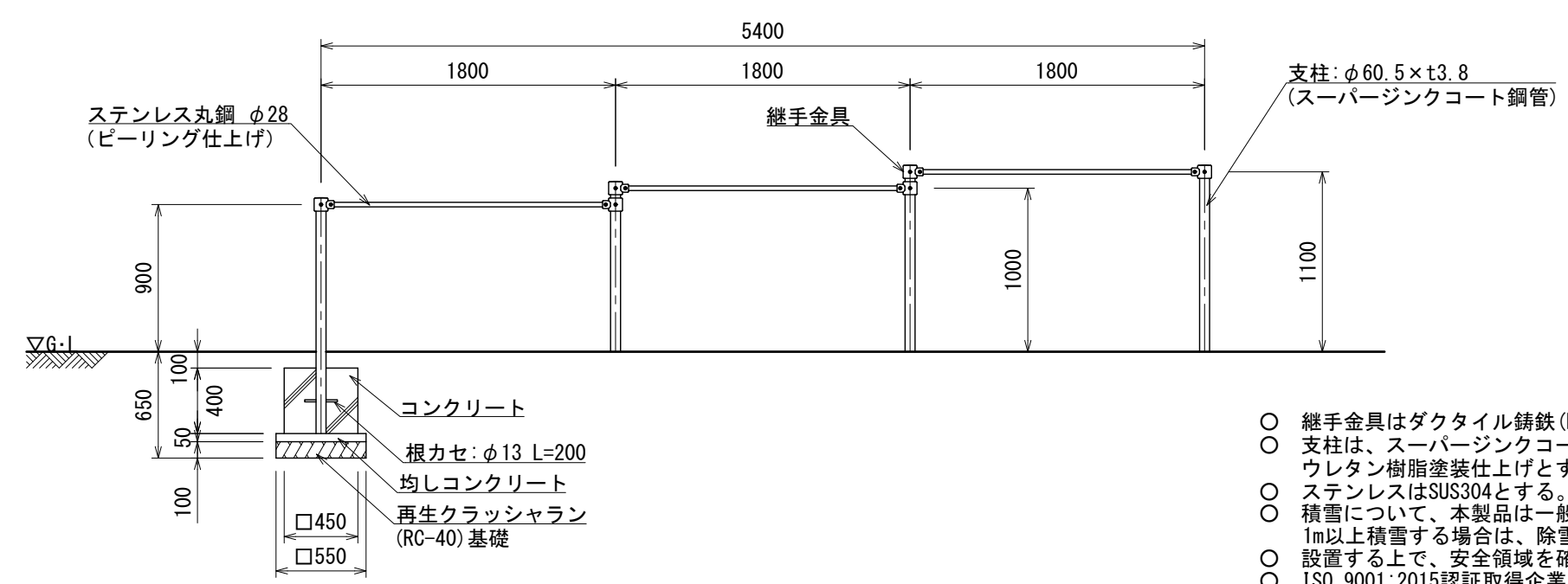
立面図
