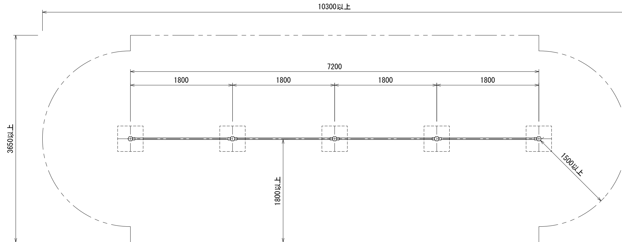
平面図
