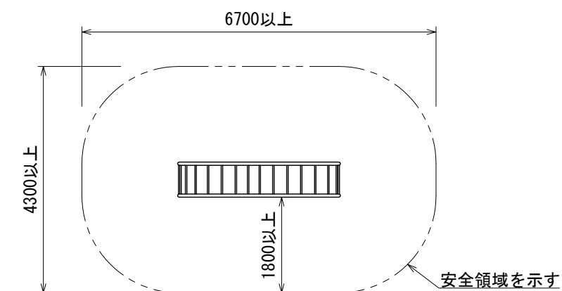
安全領域図 S=1:100
