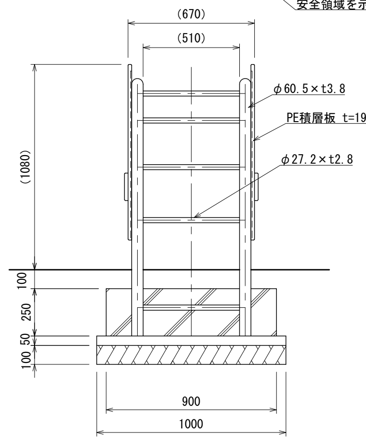
安全領域図 S=1:100
