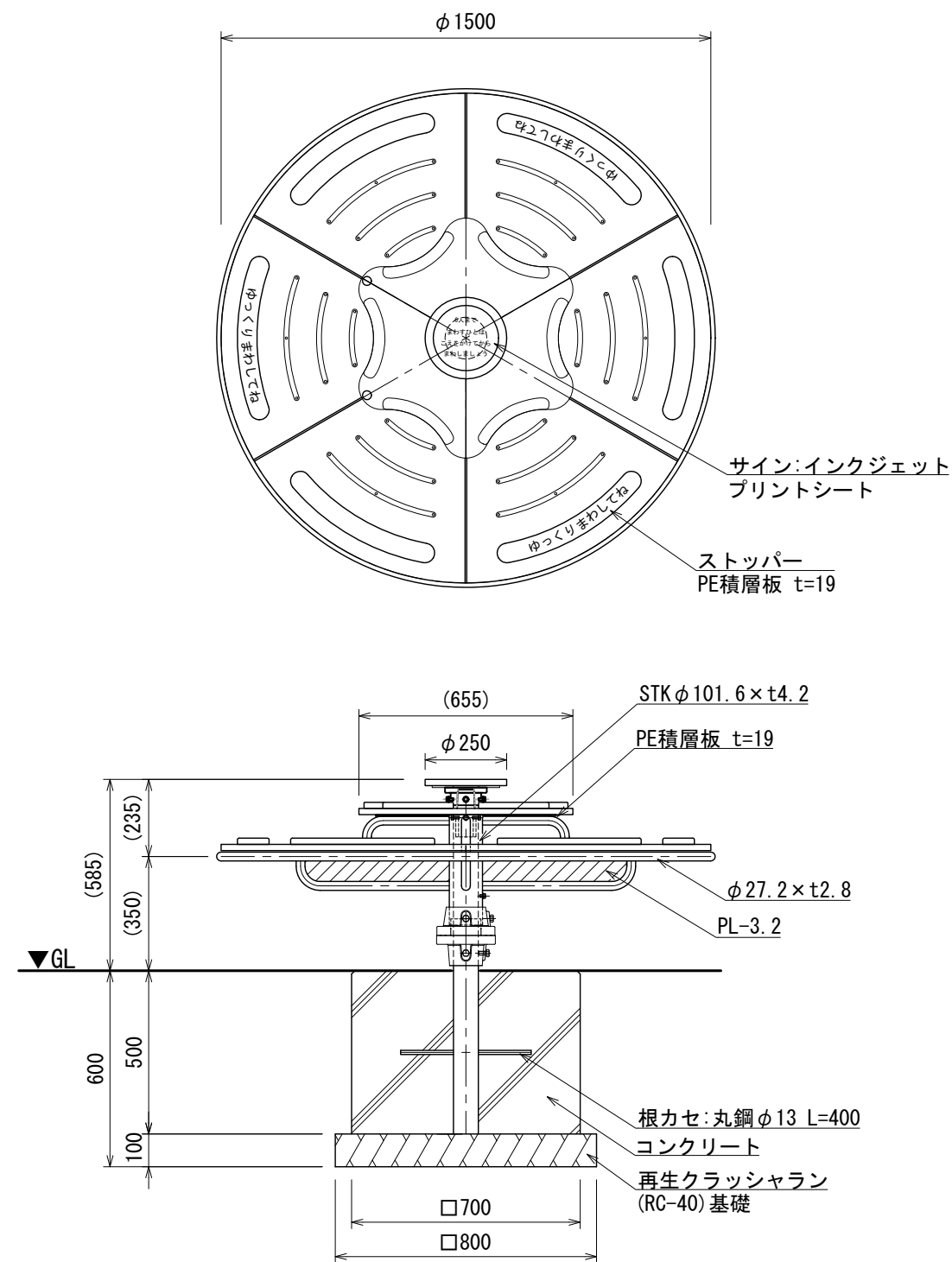
立面図
