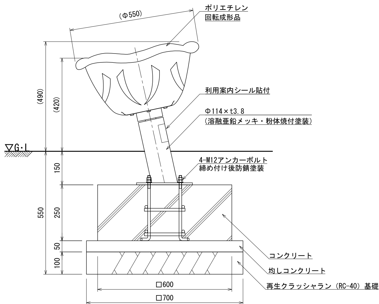
立面図
