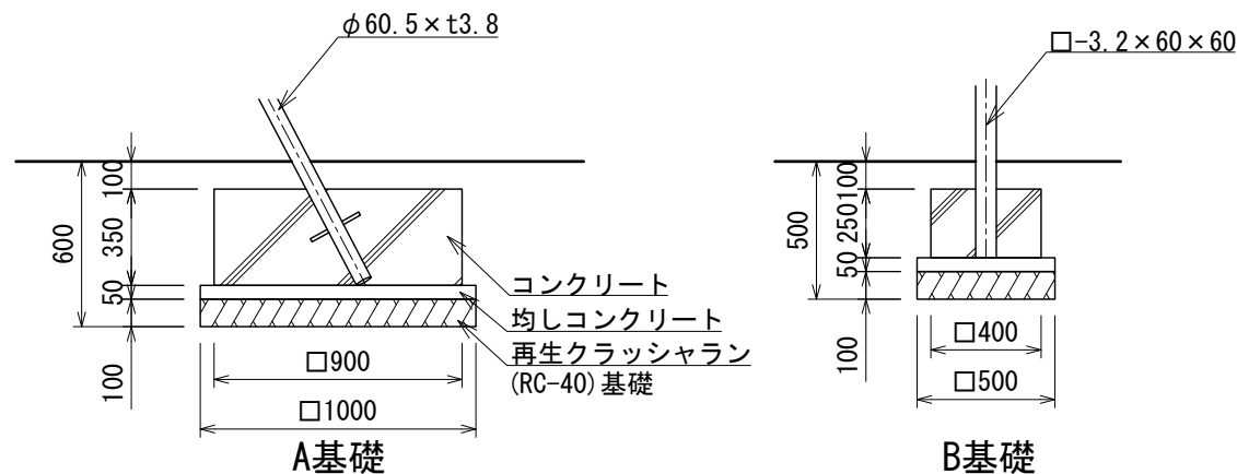
基礎詳細図 S=1:30
