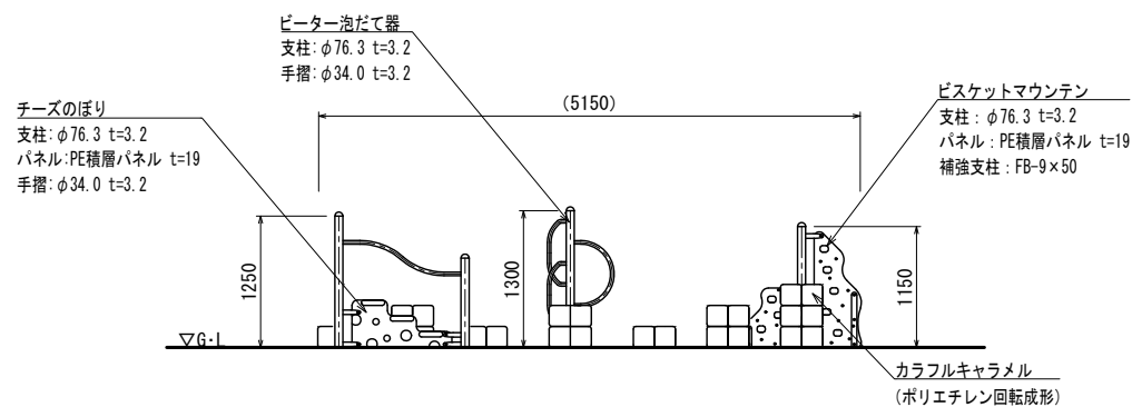
基礎詳細図 S=1:30 (A1) S=1:60 (A3)
