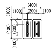
H200 (2列)
