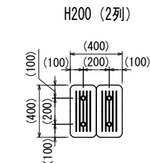
カラフルキャラメル詳細図 S=1:20 (A1) S=1:40 (A3)
