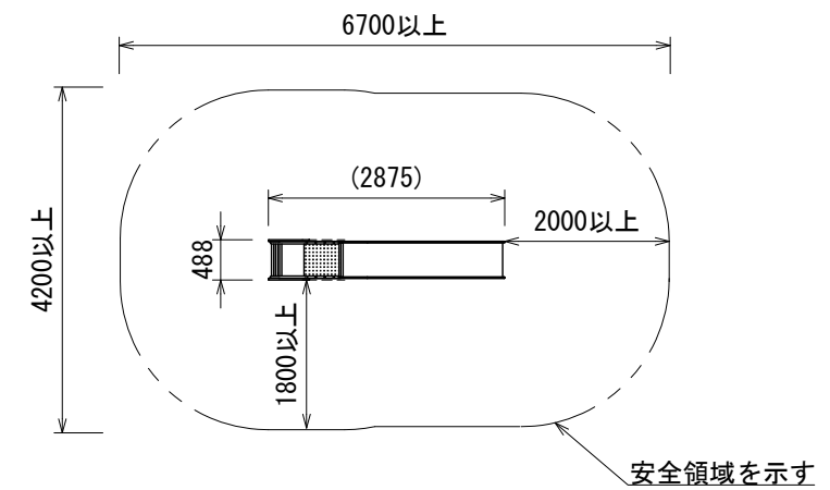
安全領域図 S=1:100
