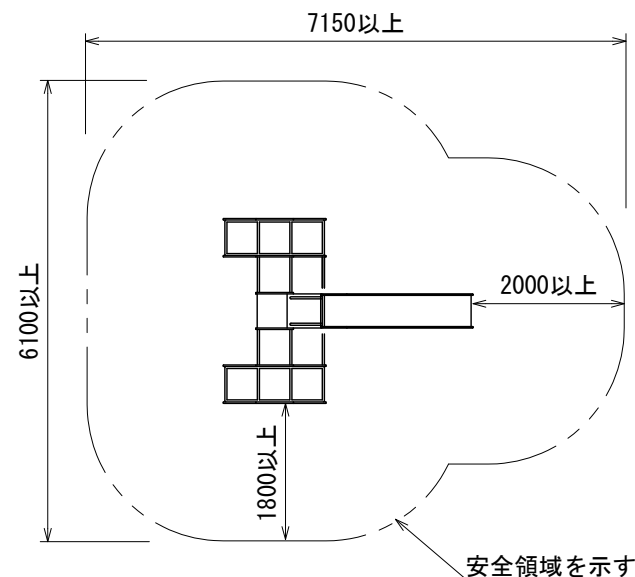
安全領域図 S=1:100
