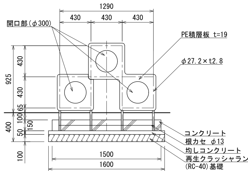
B矢视图
