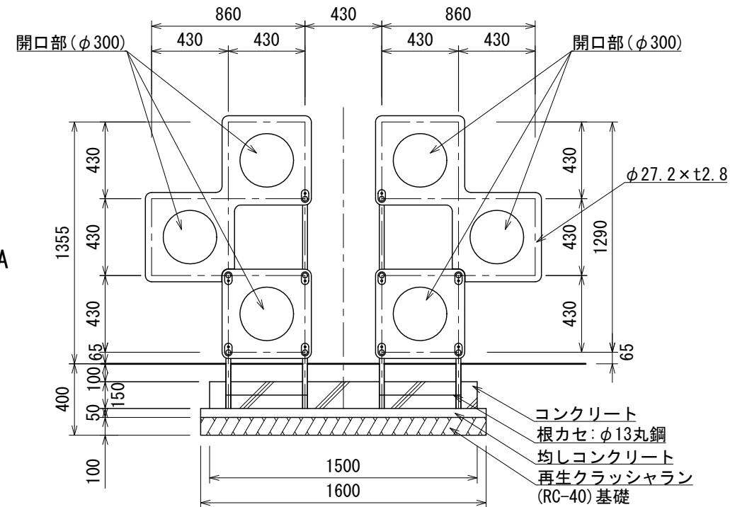
A矢视图
