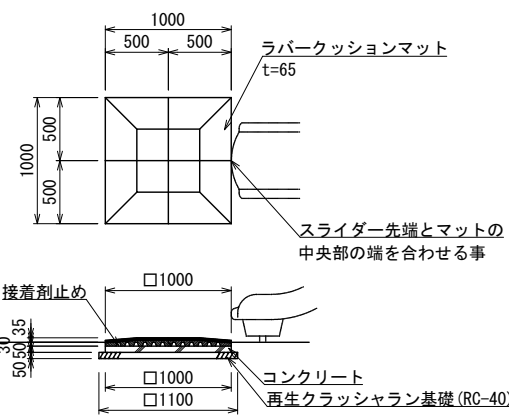
オプション ラバークッションマット詳細図 S=1:30 (A3 S=1:60) [A0-9112]
