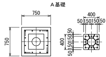
基礎詳細図 S=1:30 (A3 S=1:60)
