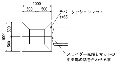
オプション ラバークッションマット詳細図 S=1:30 (A3 S=1:60) Aタイプ [A0-9112]
