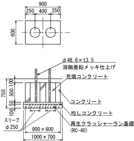
E' 基礎詳細図
