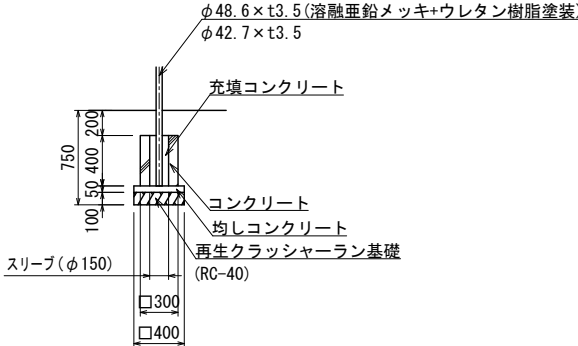
C' 1基礎詳細図
