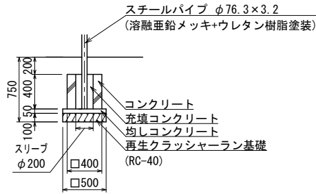
D' 1基礎詳細図
