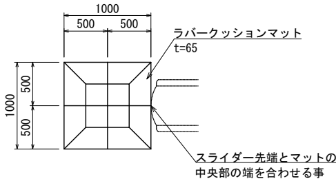
ラバークッションマット詳細図 S=1:30 (A3 S=1:60)
