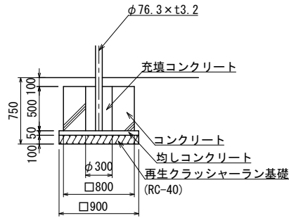
B' 1基礎詳細図
