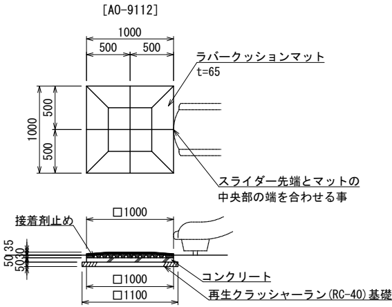
オプション ラバークッションマット詳細図
