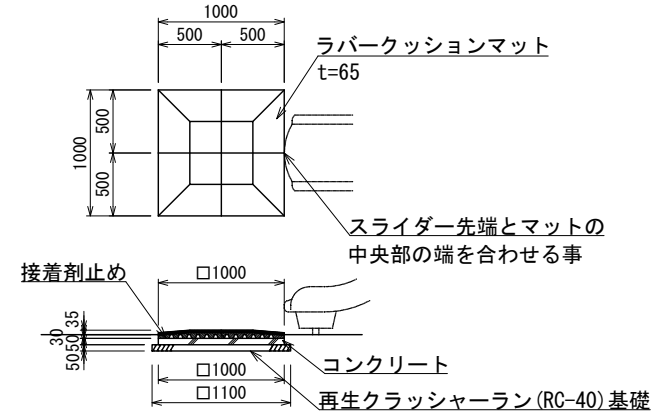
オプション ラバークッションマット詳細図 S=1:30 (A3 S=1:60) [A0-9112]
