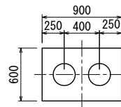
E' 基礎詳細図
