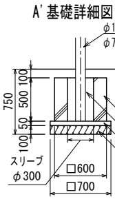
基礎詳細図 S=1:30 (A3 S=1:60)
