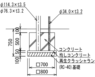
H基礎詳細図
