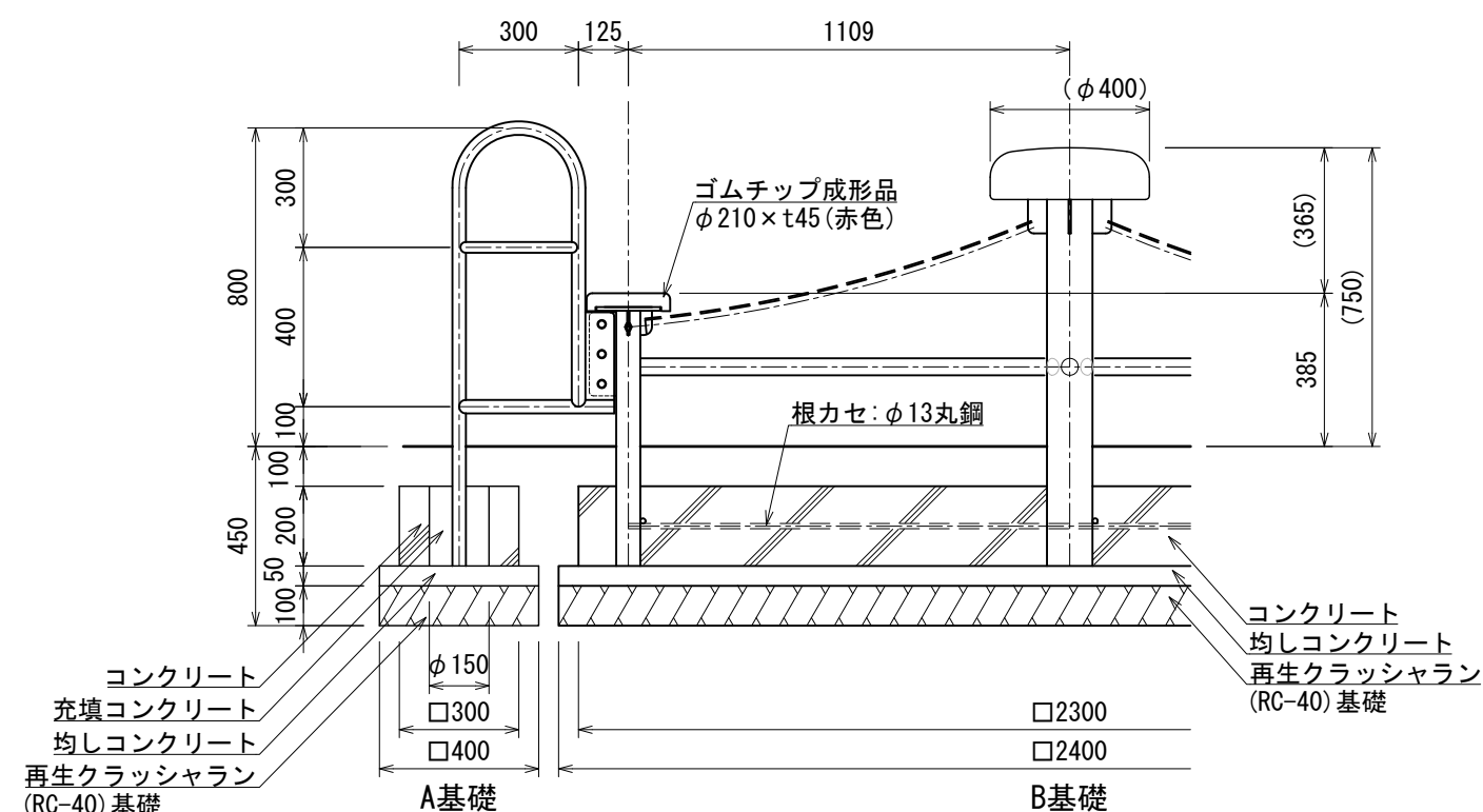
基礎詳細図 S=1:20
