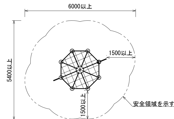
安全領域 S=1:100
