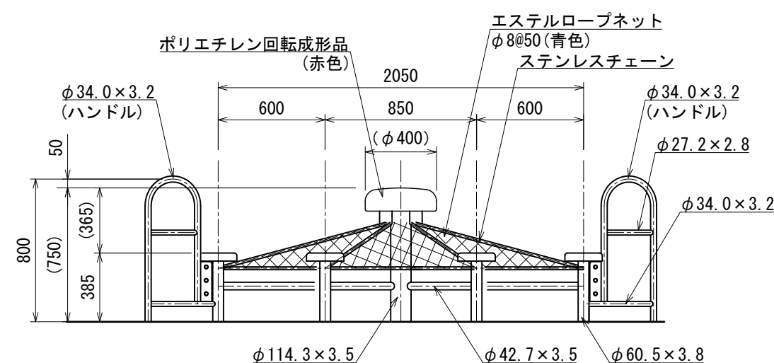
立面图
