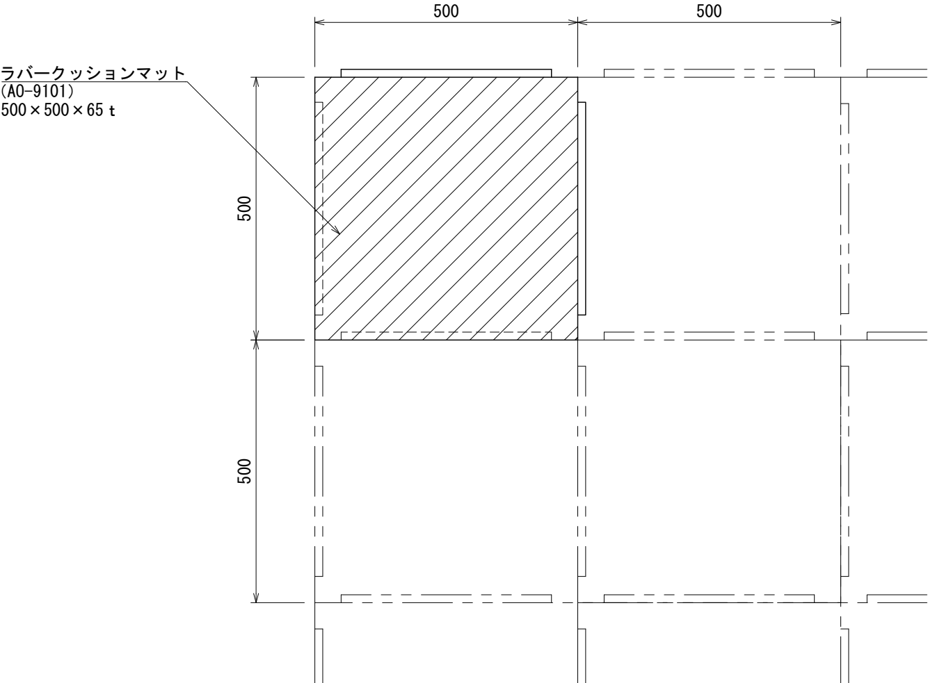
平面図
