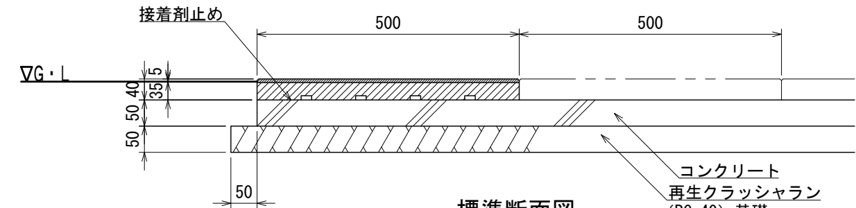
標準断面図
