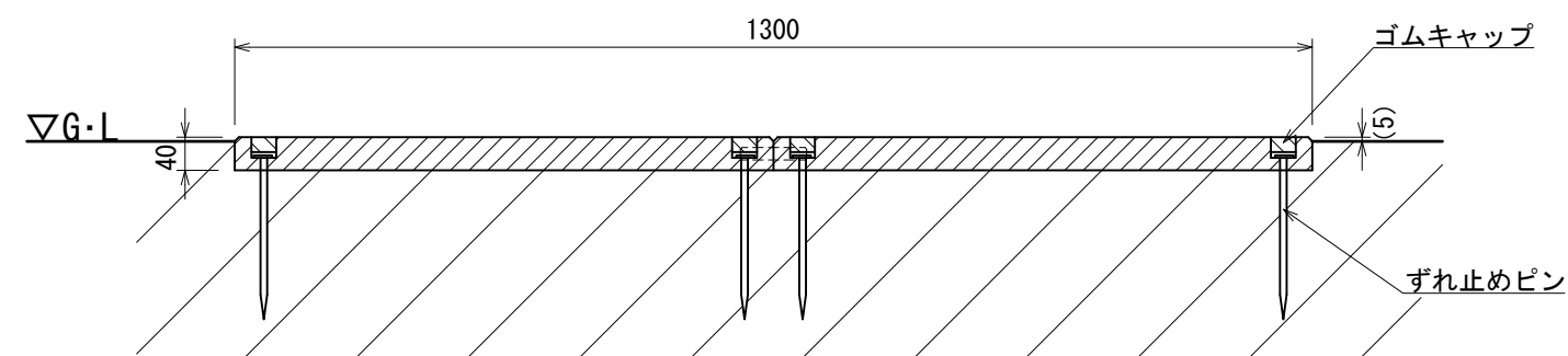
断面図
