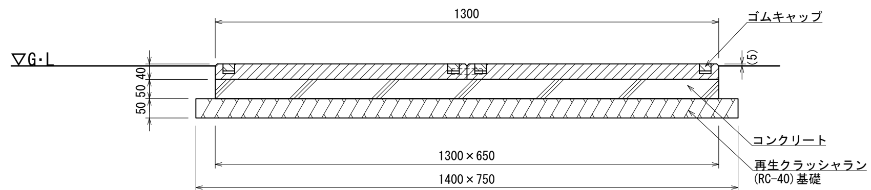
断面図
