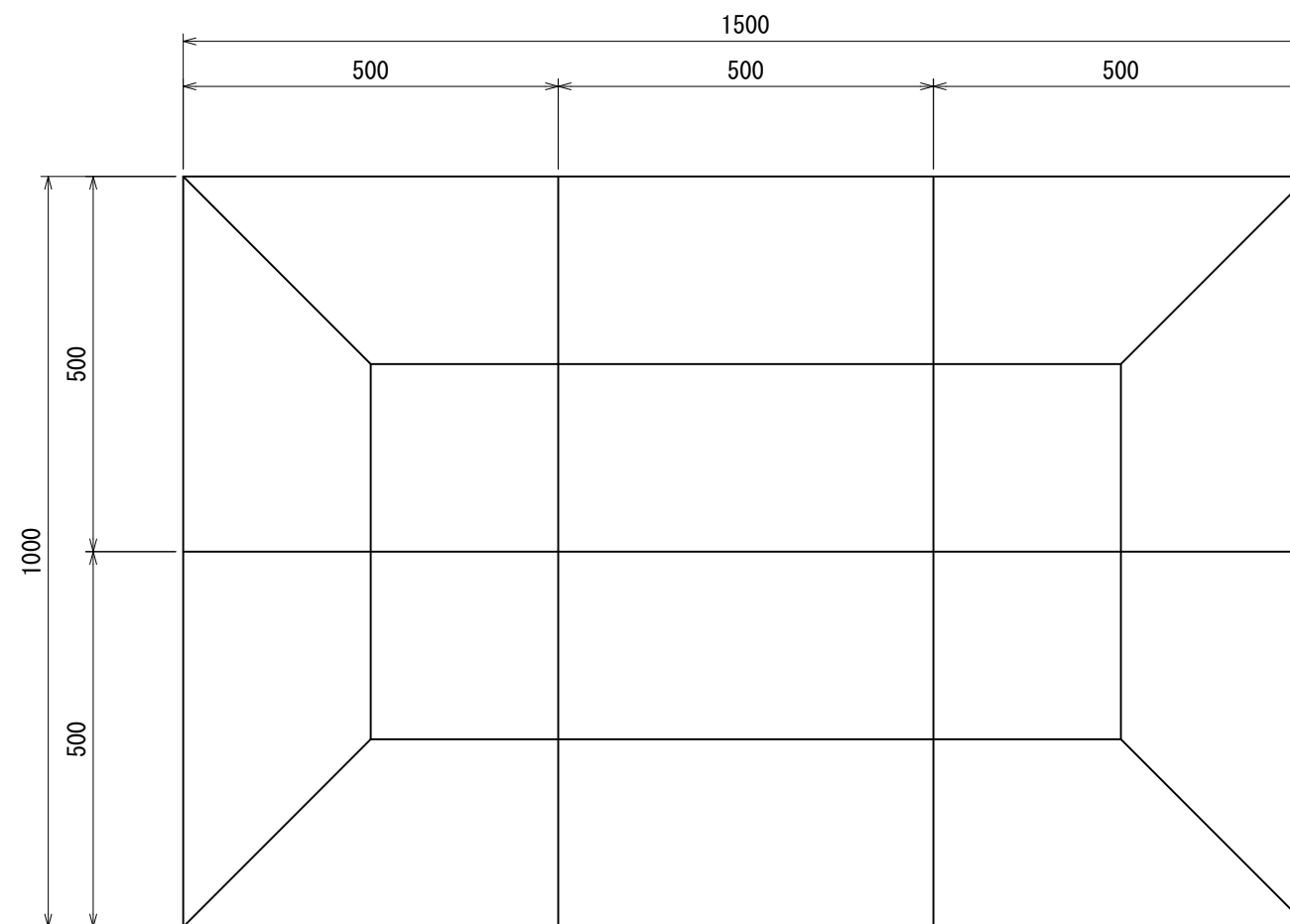
平面図
