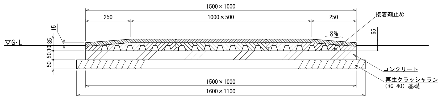
断面図
