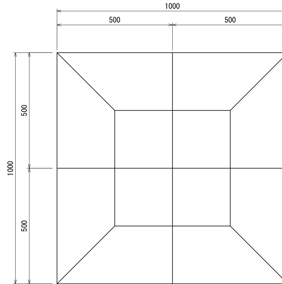
平面図
