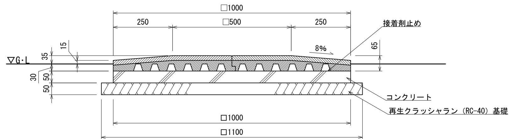
断面図
