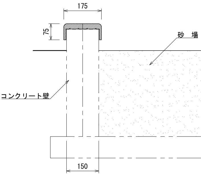
標準断面図
