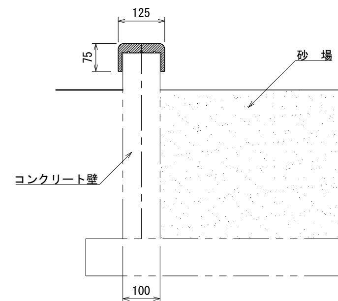
標準断面図
