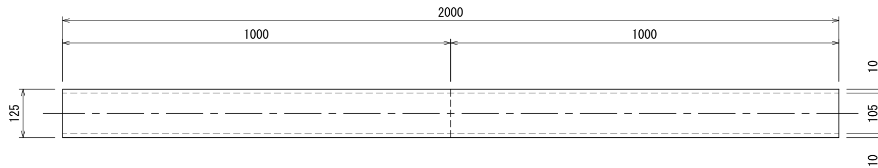
平面図
