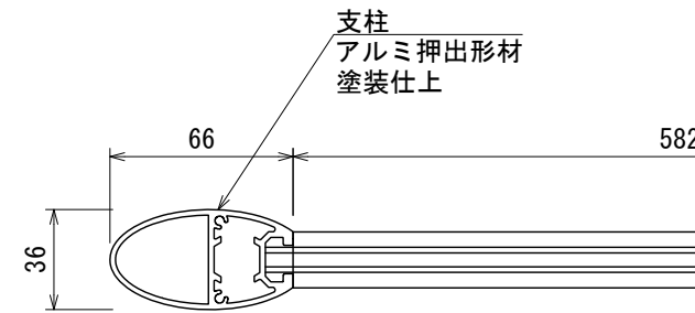
平面図 S=1:3
