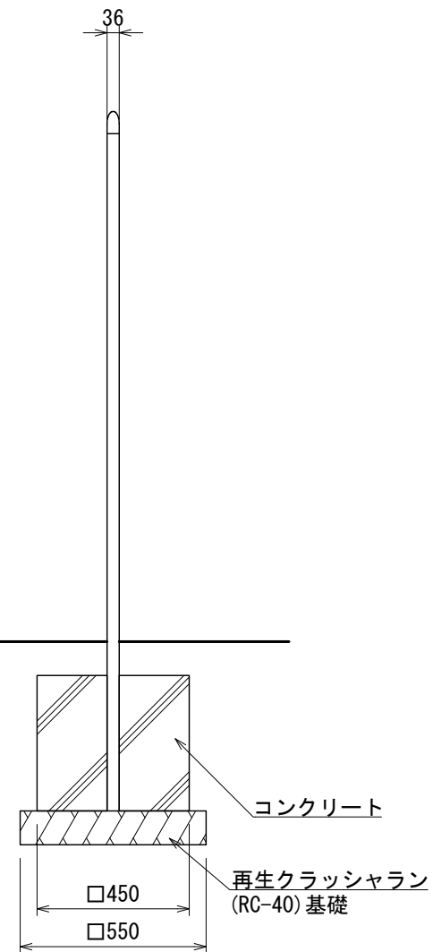
側面図
