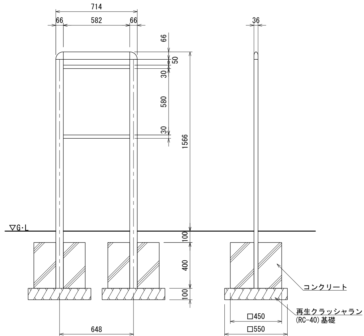
正面図
