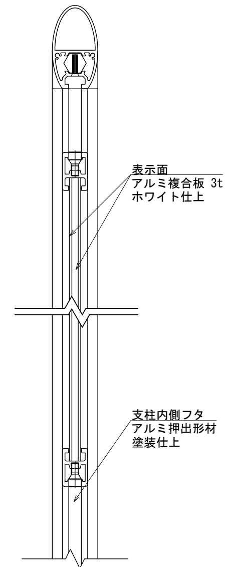
側面図 S=1:3
