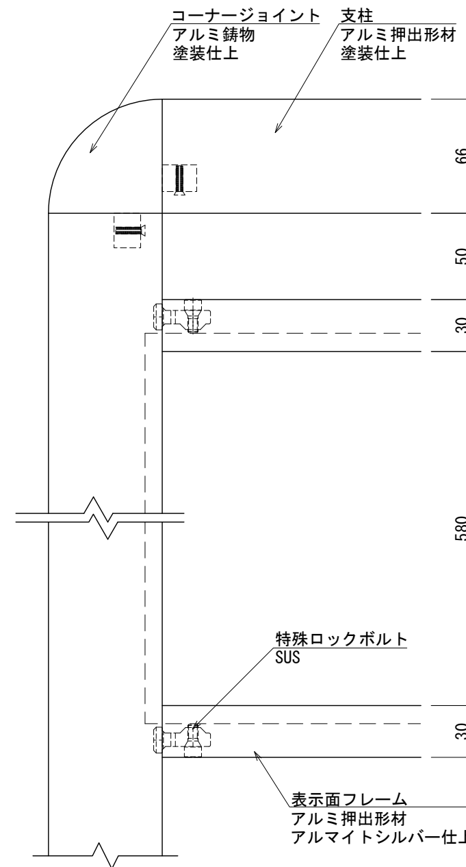
正面図 S=1:3
