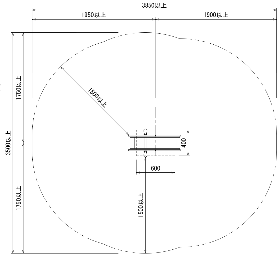
安全領域図 S=1:30
