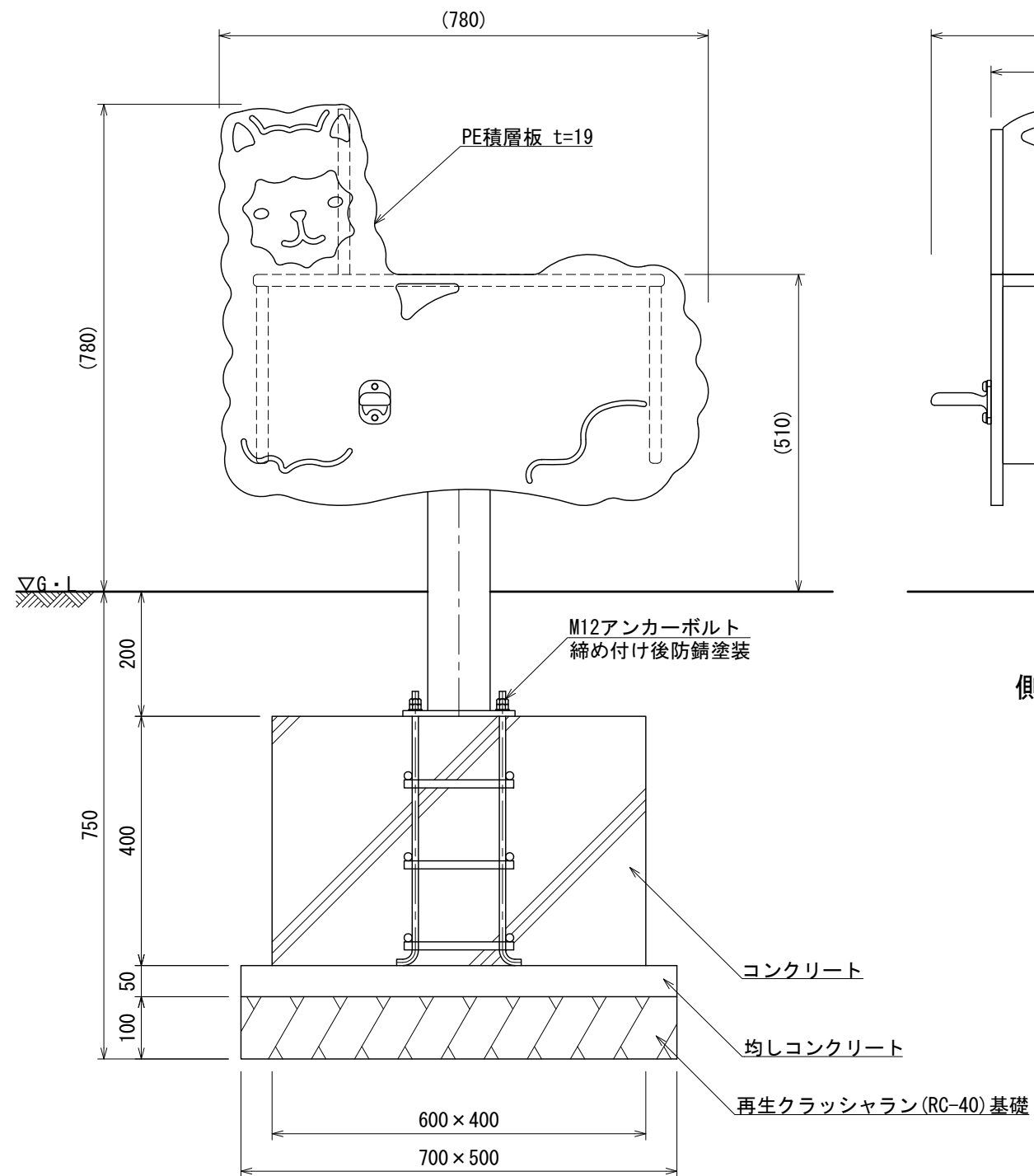
立面図
