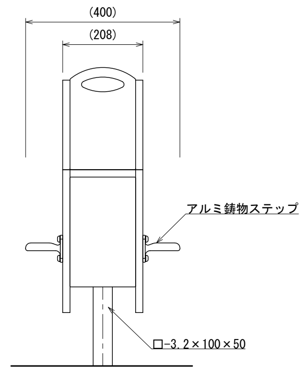
側面図
