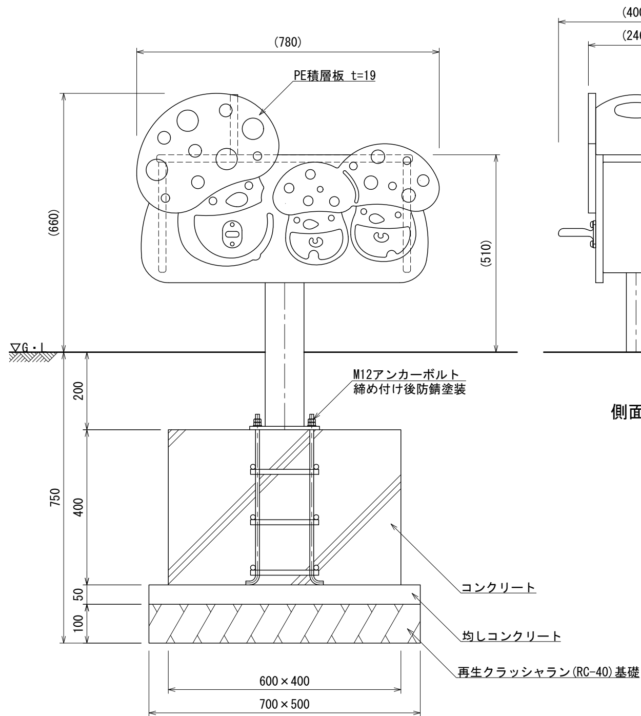
立面図
